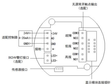
图 4-2 接线示意图
